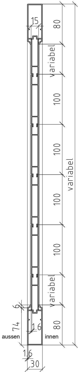
Schnitt B-B
