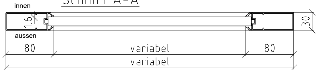
Schnitt A-A
