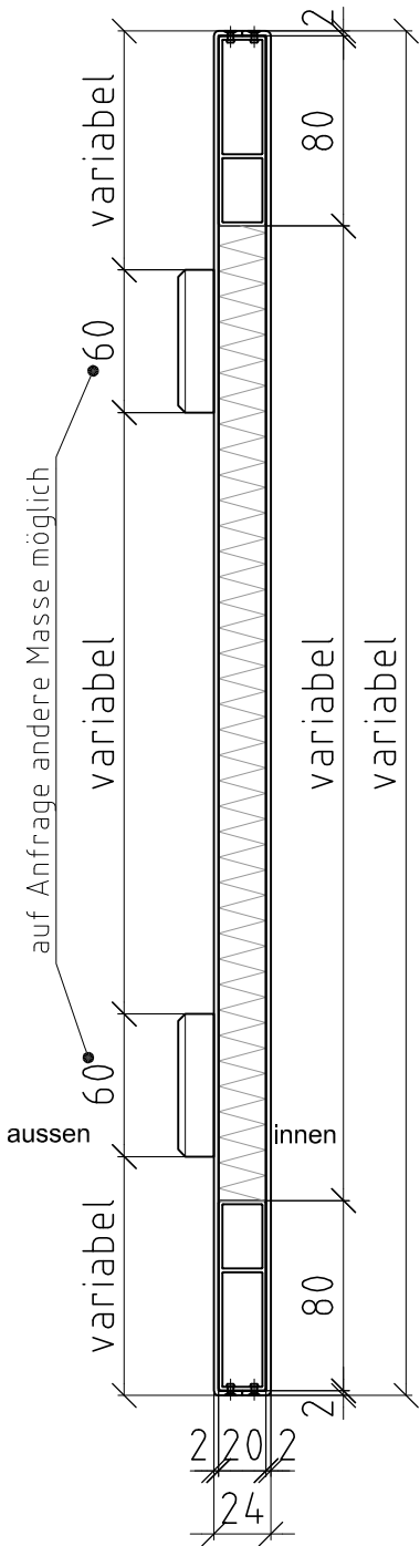
Schnitt B-B
