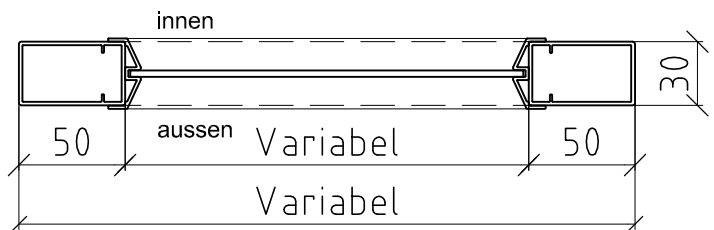
Schnitt A-A
